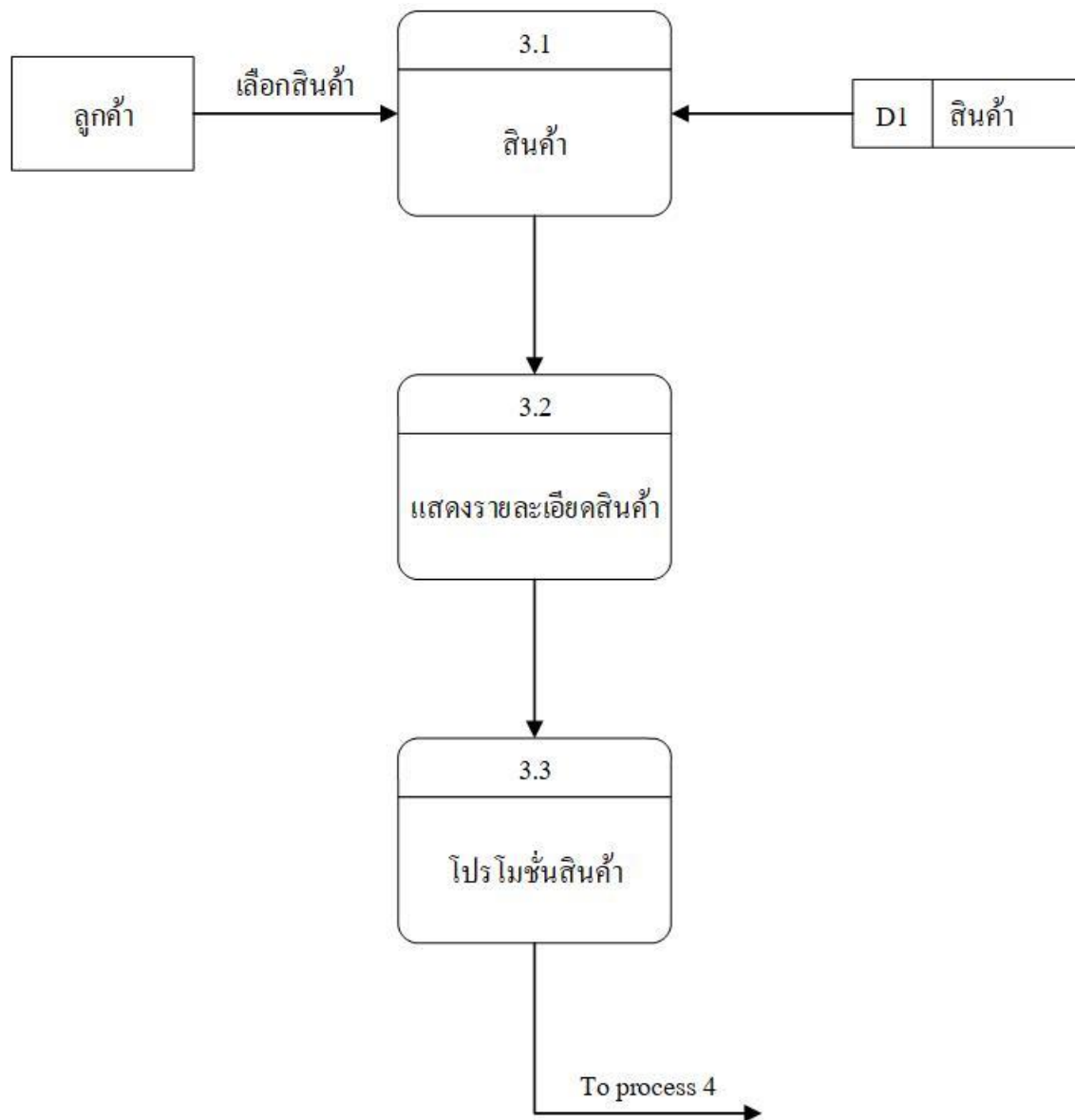
รูปที่ 3.8 Data Flow Diagram Level 1 Process 3 ระบบเลือกสินค้า
