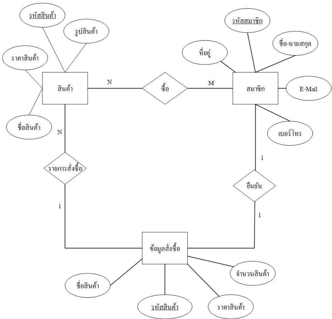
รูปที่ 3.10 E-R Diagram ระบบการขายสินค้าออนไลน์ประเภท Grilled Shrimp Shop
