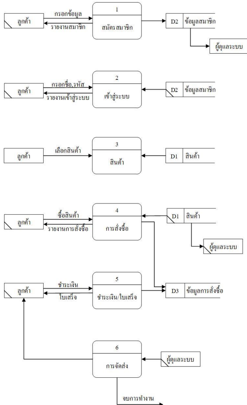
รูปที่ 3.5 Data Flow Diagram Level 0 เว็บไซต์ขายสินค้า Grilled Shrimp Shop
